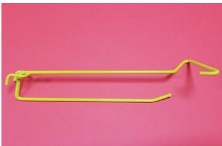
ART.192 GANCIO SINGOLO CON ASTA PORTA PREZZO, FILO DIAM.3,80-4,80 MM
