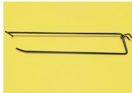
ART.190 GANCIO SINGOLO CON ASTA PORTAPREZZO ,ATTACCO ALLA RETE CON PIASTRINA ,FILO DIAM.3,80-4,80
